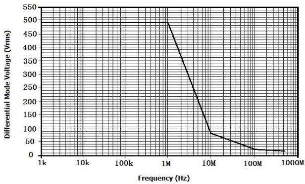
图 1 DPX6070B 最大差模电压 VS 频率
